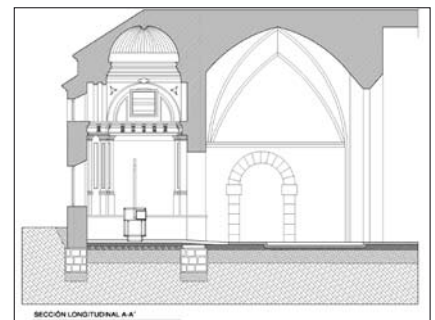
Sección Longitudinal Estado Final
