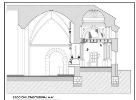
Sección Longitudinal Estado Previo
